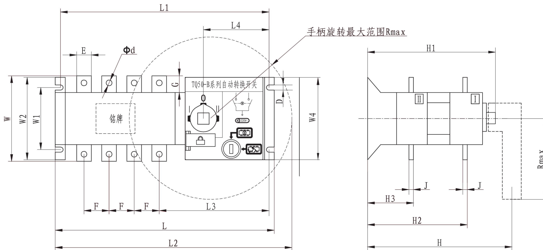
图1 壳架等级100A~630A开关示意图
